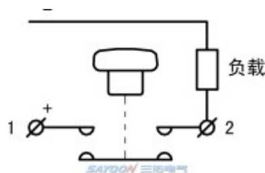
一路 1、2为触点接线端
