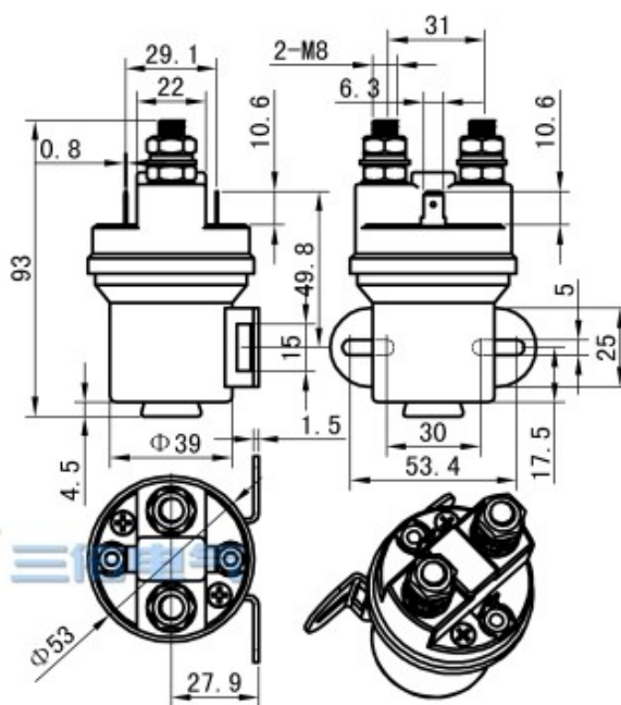
MP 平支架 插片接线 MP Flat support, Spade terminals
