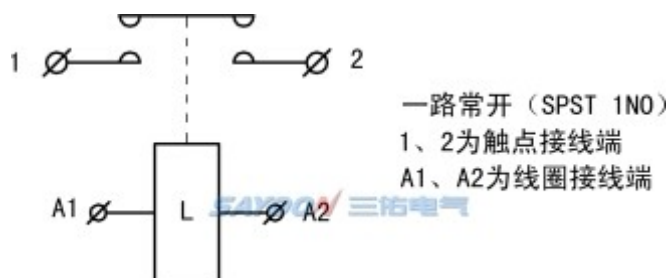
线路原理图
